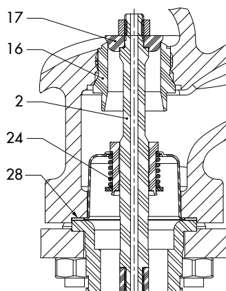
wykonanie standardowe, średnica nominalna od DN 15 do DN 25
