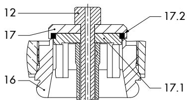
wykonanie z grzybem z uszczelnieniem miękkim
