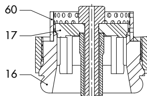
wykonanie z rozdzielaczem strumienia
