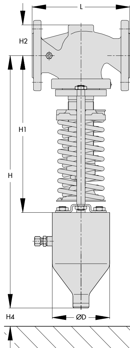
Type 41-73 avec servomoteur à soufflet
