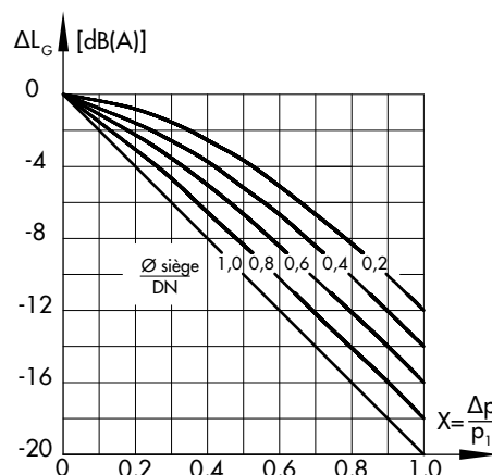
Fig. 3 : Diagramme \cdot \Delta L_G pour gaz et vapeurs
