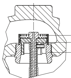
Clapet à étanchéité métallique, avec répartiteur de flux ST1
